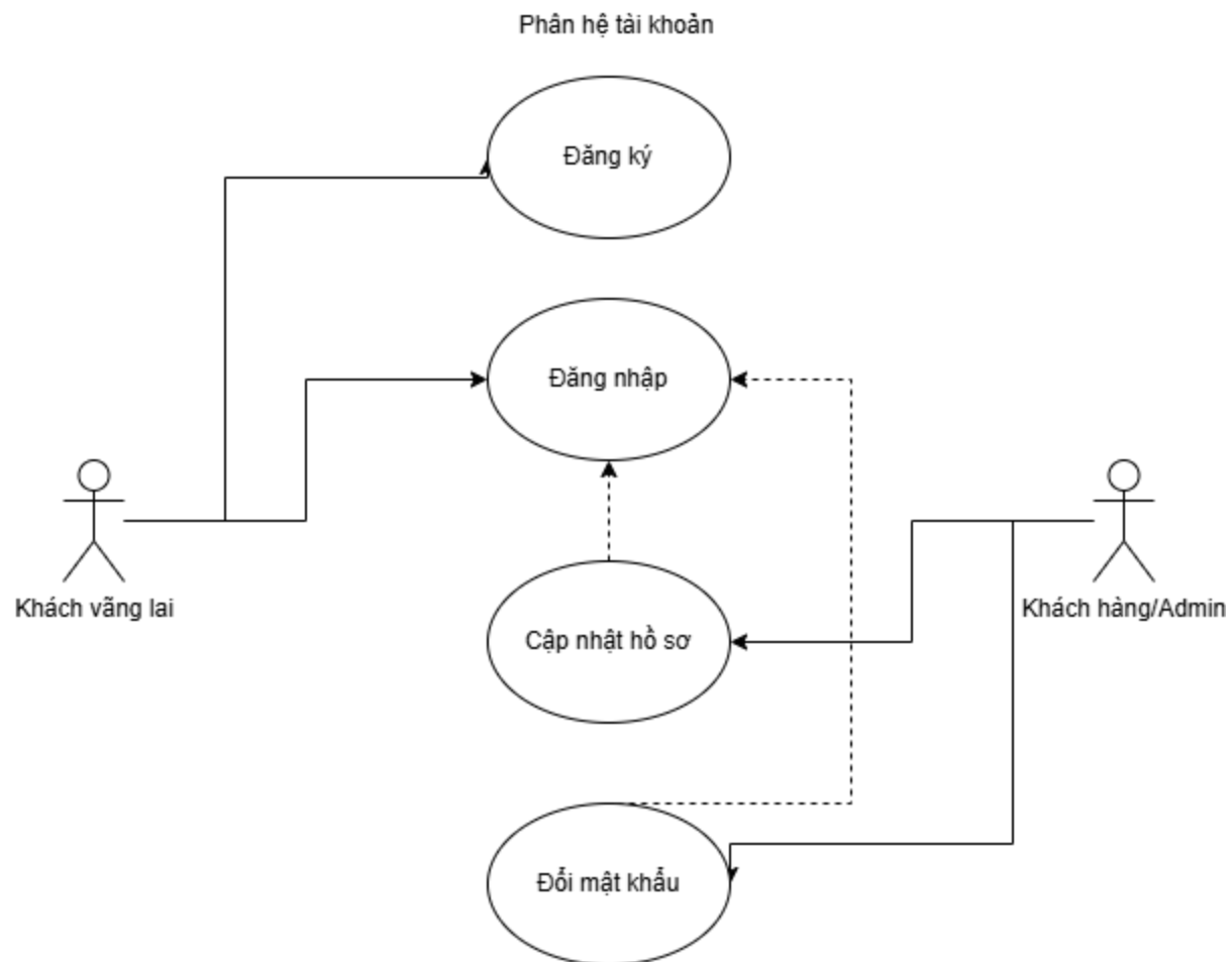
Use Case Phân hệ Tài khoản
