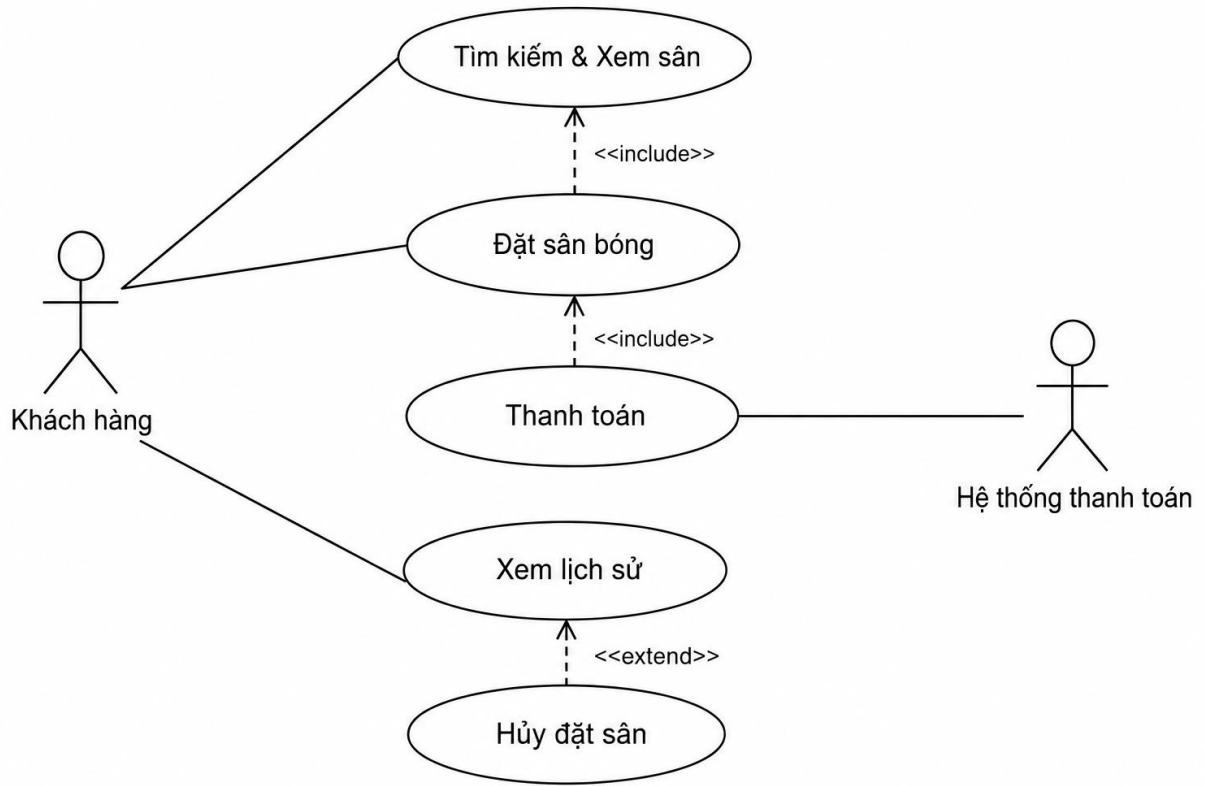
Sơ đồ Use Case chi tiết theo phân hệ
