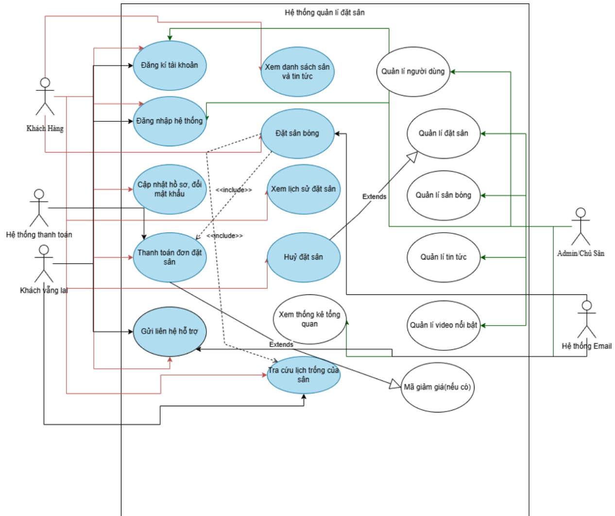
Biểu đồ User Case
